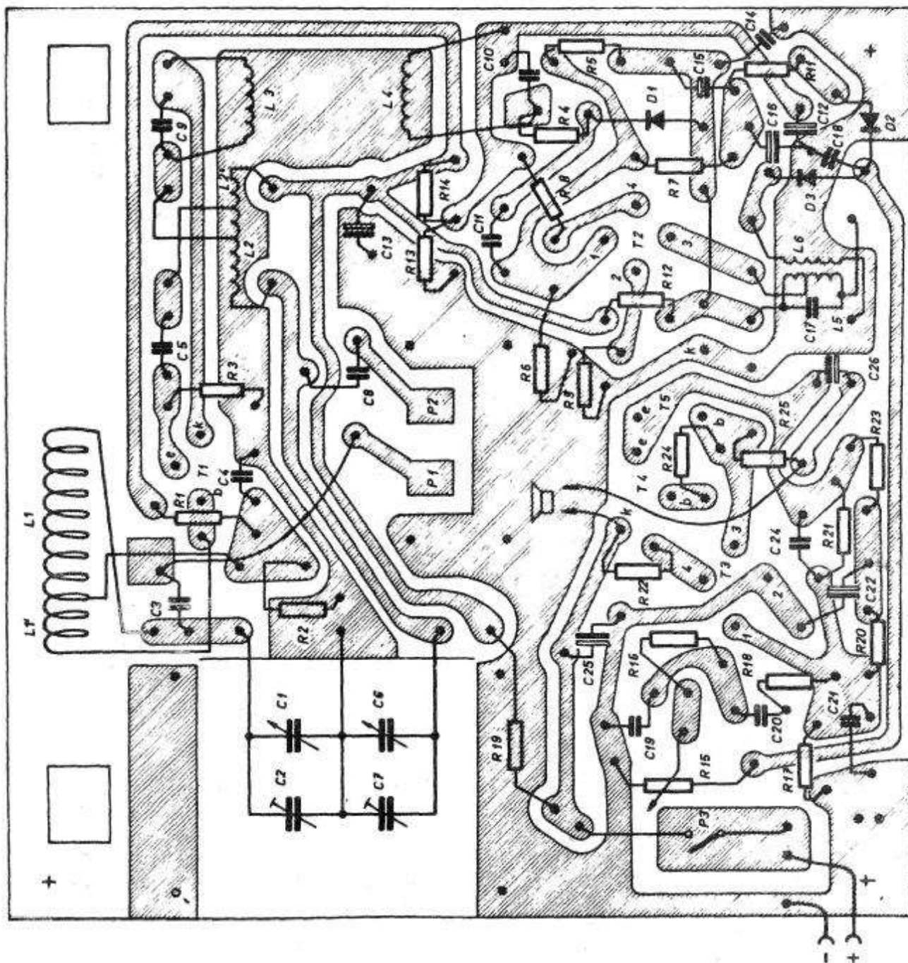
Zapojení přijímače - pohled ze strany plošných spojů
